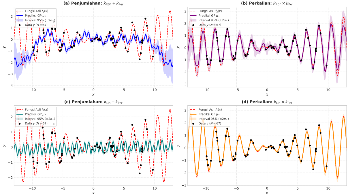
Gambar 3: Hasil fitting Gaussian Process Regression pada fungsi asli f_2(x) (36): (a) k_{\text{RBF}} + k_{\text{Per}} ; (b) k_{\text{RBF}} \times k_{\text{Per}} ; (c) k_{\text{Lin}} + k_{\text{Per}} ; (d) k_{\text{Lin}} \times k_{\text{Per}} .
